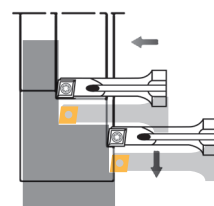
Stelo in acciaio _ Stahlschaft _ Steelshank
