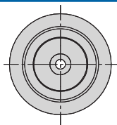
HSK-F DIN 69 893 Section 1 Forme F, l'usinage grande vitesse
