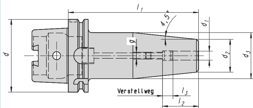
Shrink chuck InduTerm DIN 69 893-1 HSK-A long version
